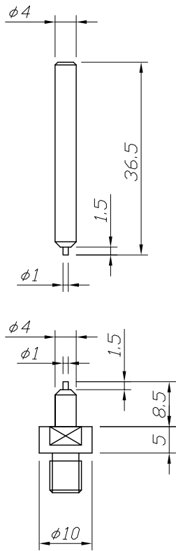
タングステン電極 KTH-DK12
