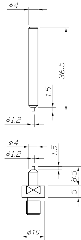
タングステン電極 KTH-DK13
